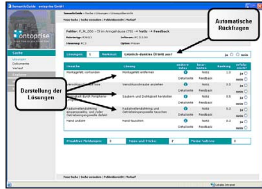
Abbildung 2: Lösungsermittlung
