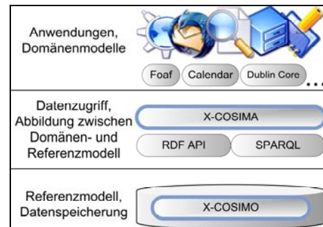
Abbildung 6: X-COSIM Architektur
