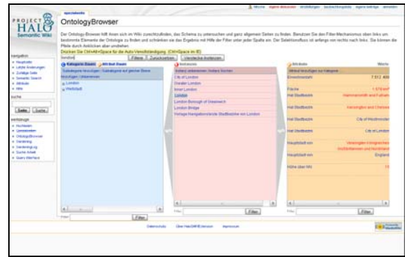
Abbildung 5: Ontologie-Browser
